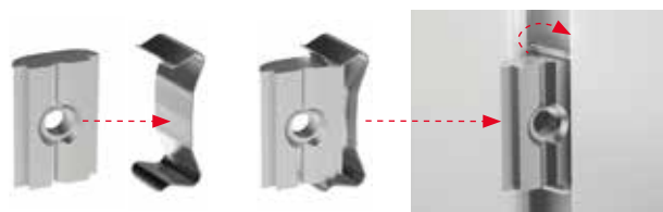
Tacos de corredera basculantes, para sujeción VESA ATPH-IP
