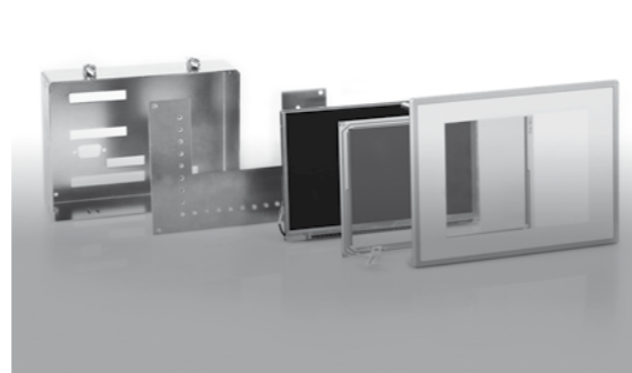
Eingabeeinheiten: Touchintegration
