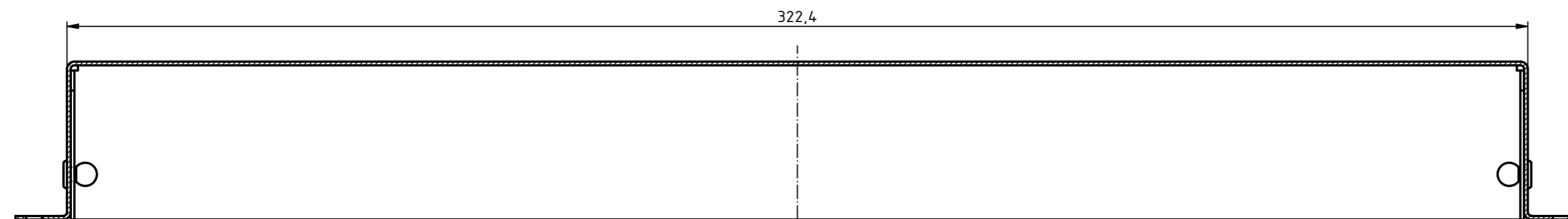
B-B ( 1 : 1 )
