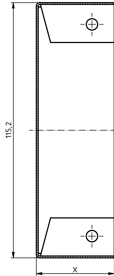
A-A ( 1 : 1 )
