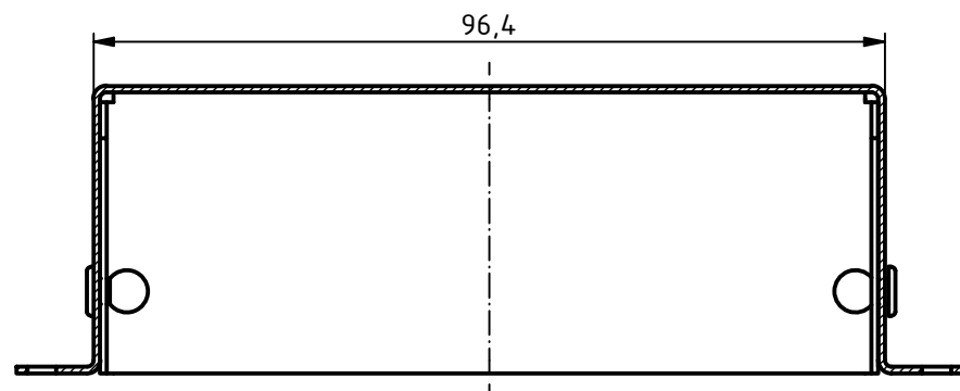
B-B ( 1 : 1 )
