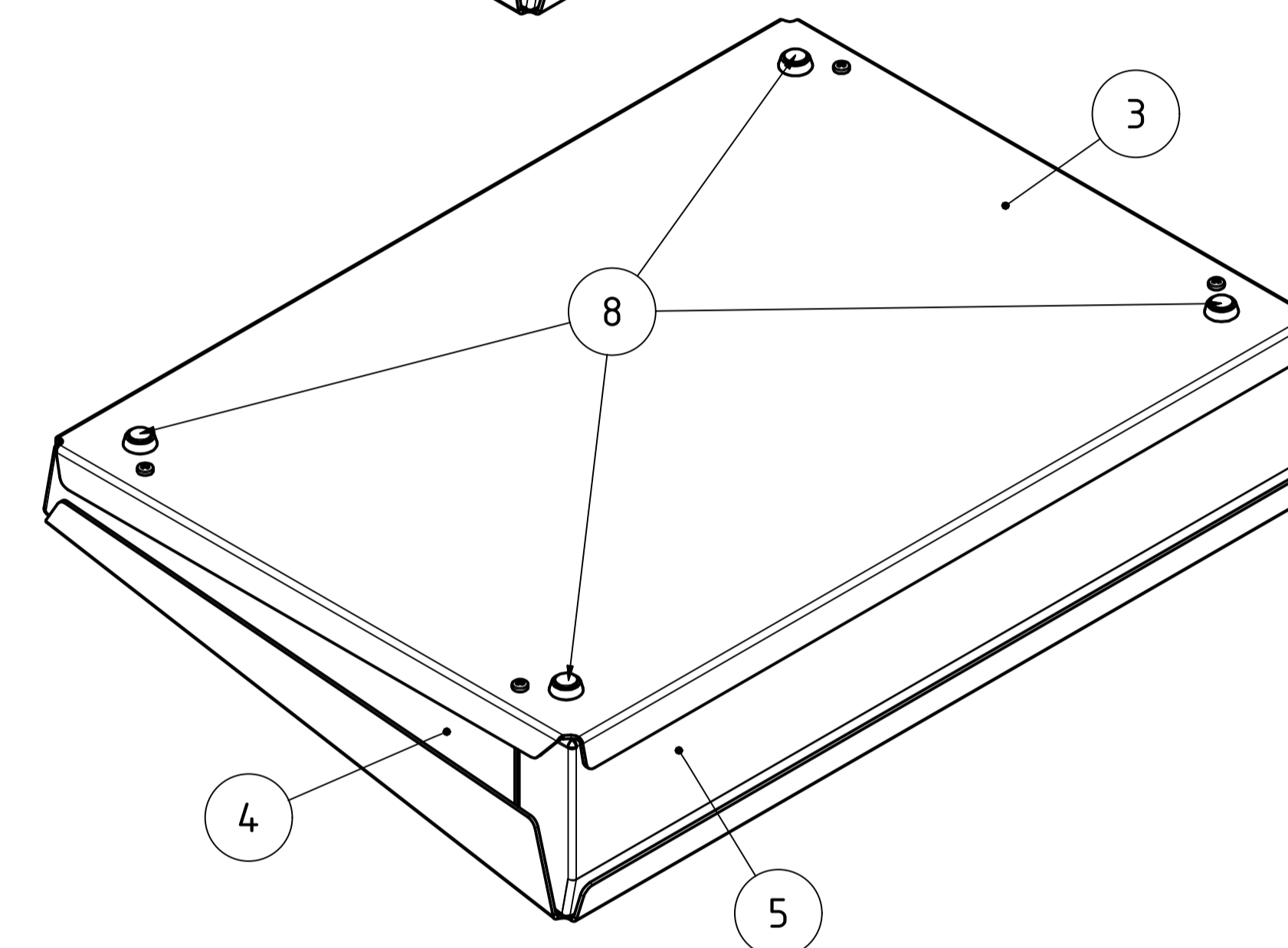
ISO-Ansicht / ISO-View ( 1:2 )
