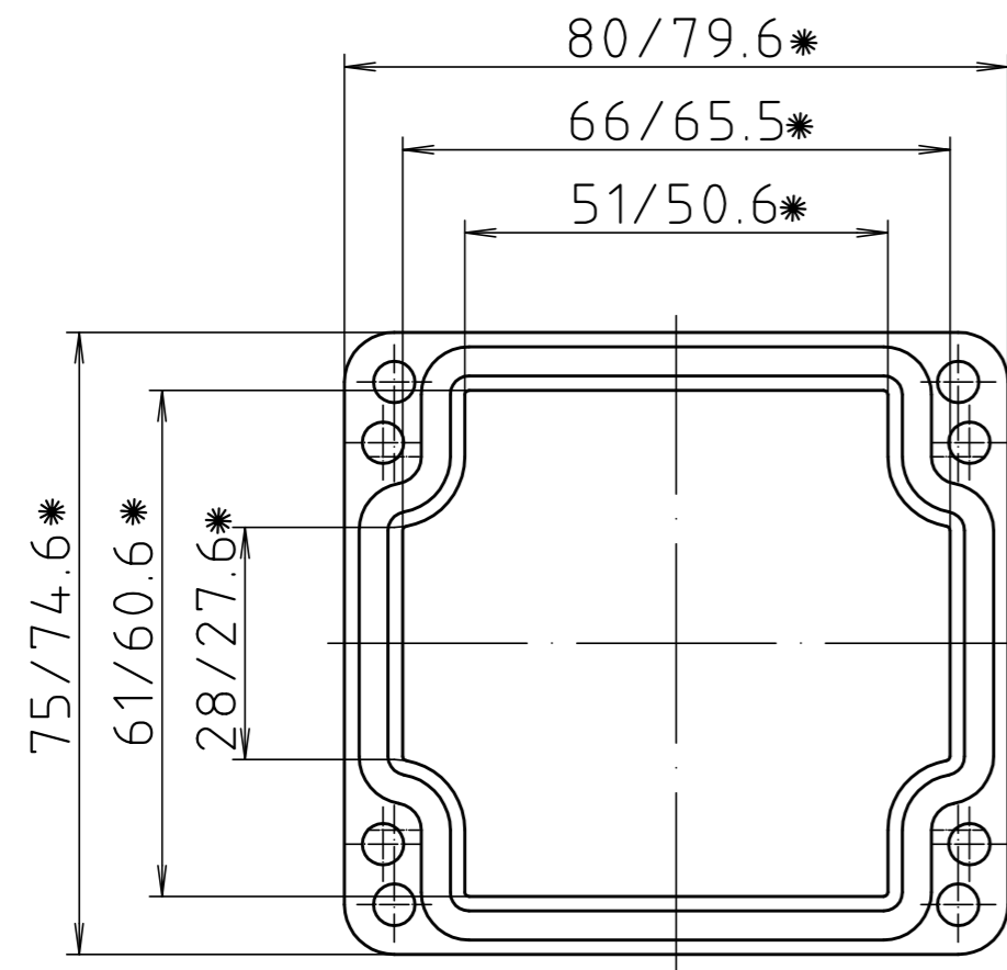
Deckel/ lid
