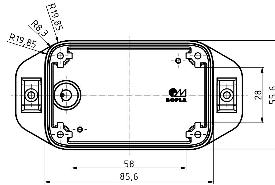
UT mit montierter Dichtung Base with mounted seal
