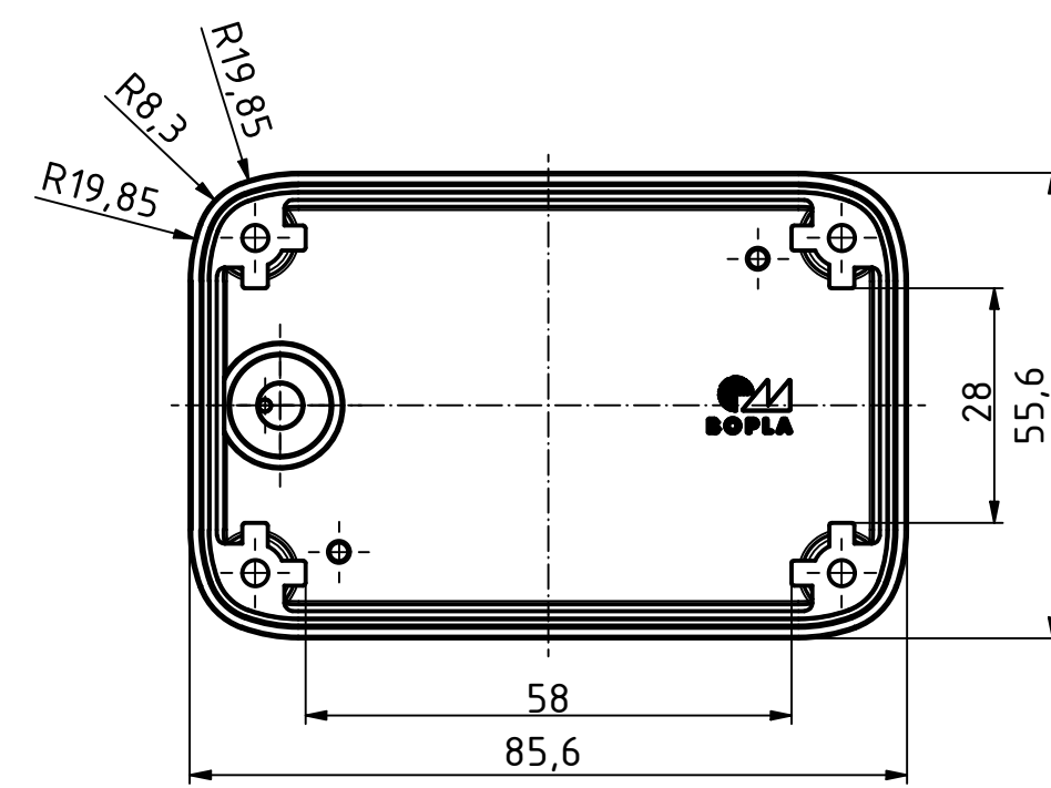
UT mit montierter Dichtung Base with mounted seal
