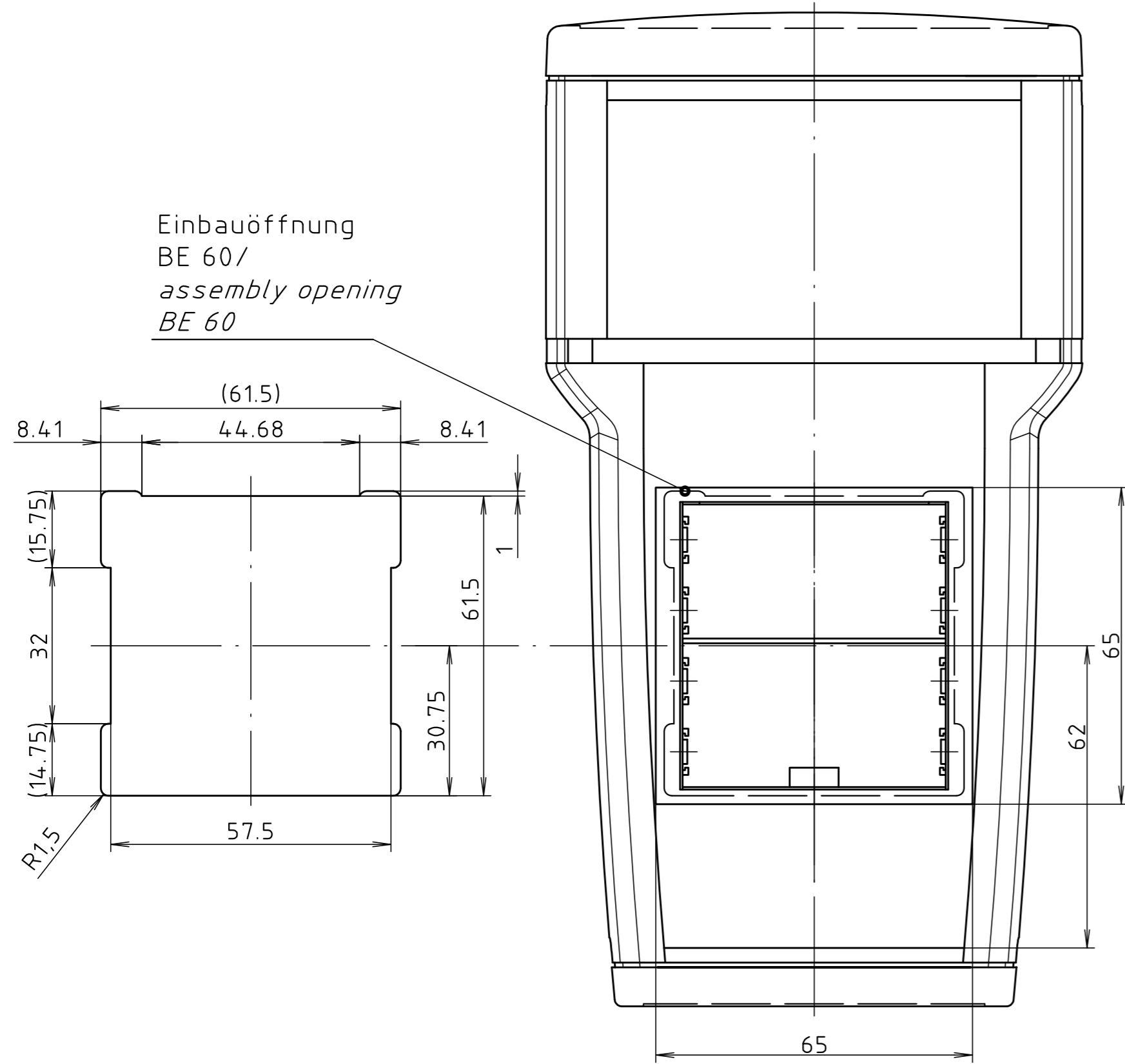
ohne Batteriefachdeckel dargestellt/ view without compartment lid
