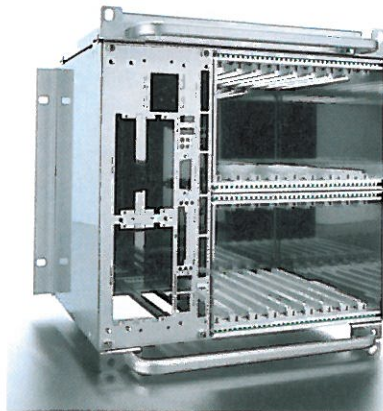
Hartmann Elektronik, der Spezialist für Backplanes bietet 19" Plattformen in EMV-Ausführung mit montierten Backplanes an.
